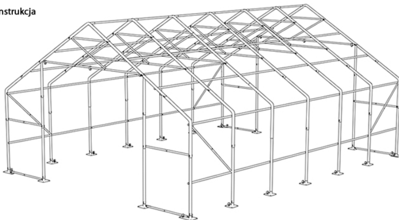
Złożona konstrukcja 9x16 (połączenie dwóch konstrukcji 9x8)
